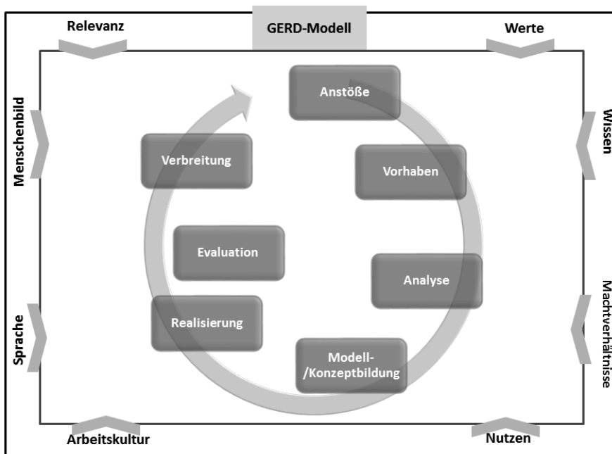
Abbildung 1: Das GERD-Modell
